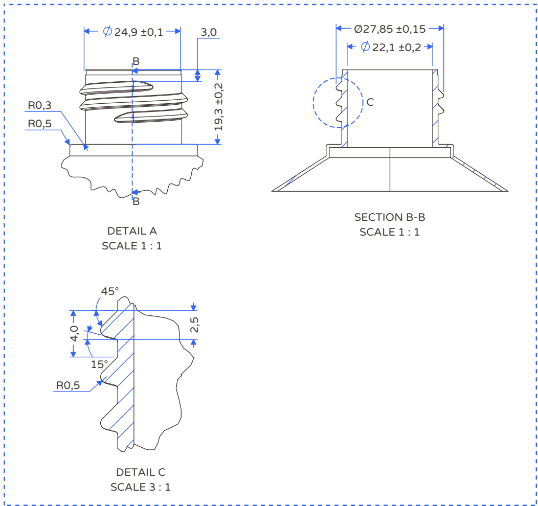
Neck : 28/410 - RND.0100
